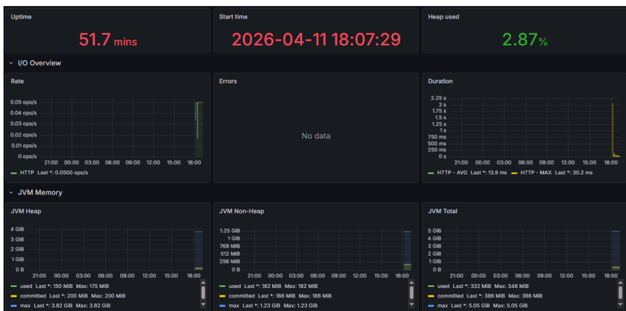
Рисунок 5.4 – Панель с метриками микросервисов в Grafana
